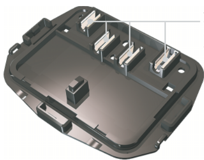
Anschluss für Flachbandleiter 4 – 8mm × 0,15 – 0,5mm Connections for bus ribbons 4 – 8mm × 0,15 – 0,5mm
