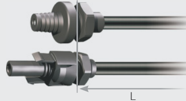
Aufbaudosenbuchse Female panel receptacle
